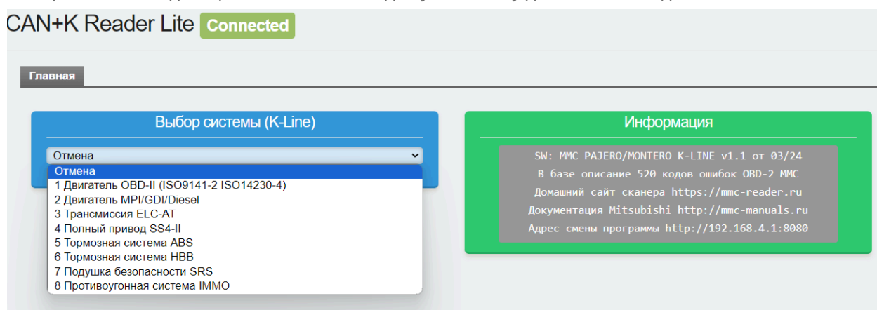
Рис.3 Выпадающий список систем
