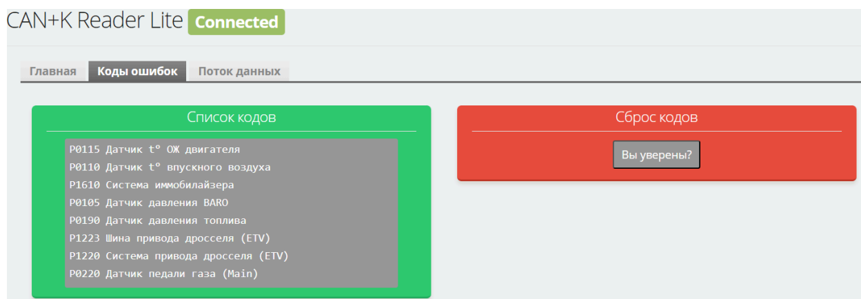
Рис.5 Просмотр и сброс кодов ошибок
