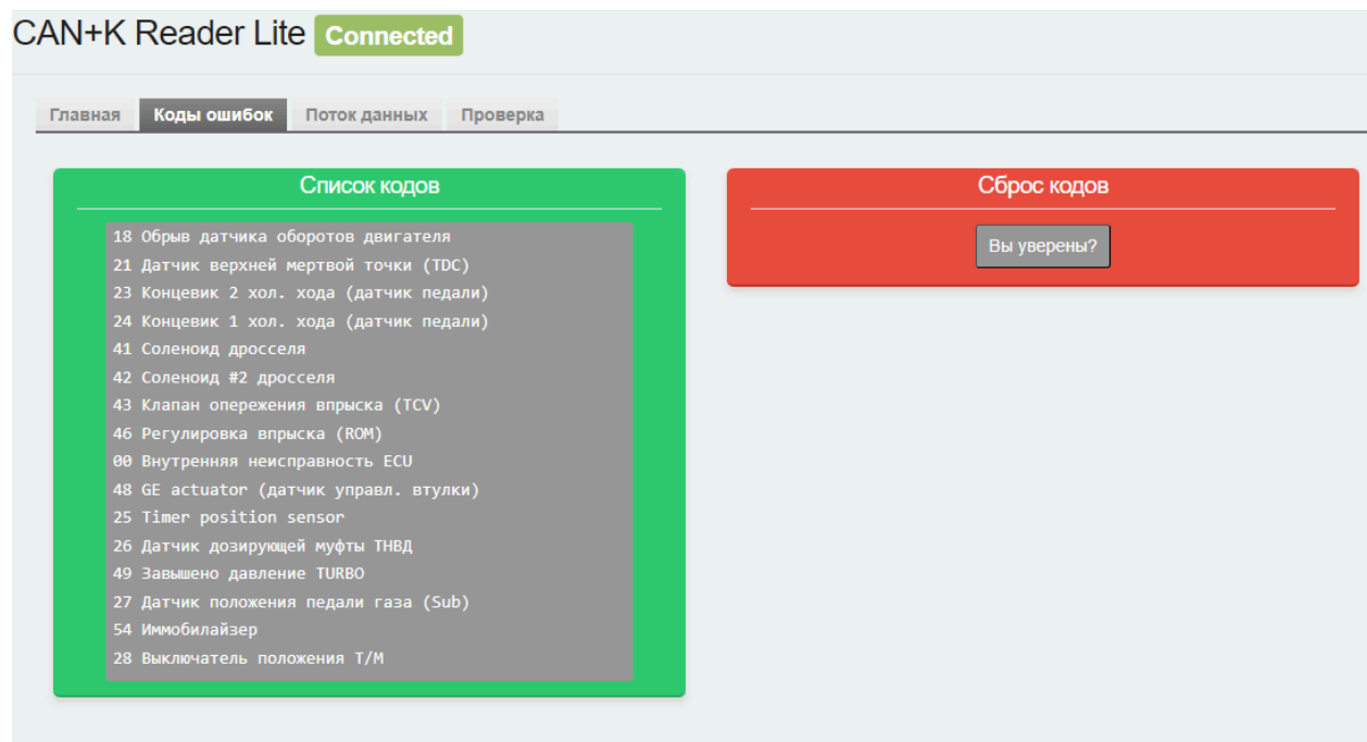
Рис.9 Диагностика с кодами ошибок по заводскому протоколу
